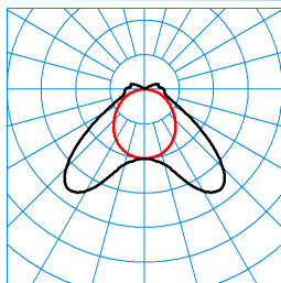
AragF 15 PVW 80-840 ETDD +HFSB LV PC TX112867
