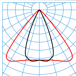
7651 Grado 30-830 J21 ET L37 05 (150) TX783520
