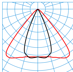
7651 Grado 30-830 J21 ET L37 05 (225) TX768934
