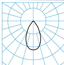
Amatris G3 C04 HR 1400-840 01 TX374673
