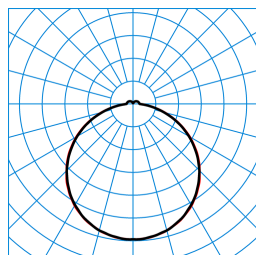
Olisq QWD2 DW 35-830 ET IK + Olisq QWD2 ZDR 1/2 03 TX462301
