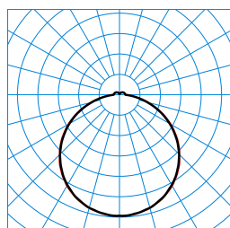
Olisq QWD2 DW 35-830 ET IK + Olisq QWD2 ZDR 1/2 05 TX461566
