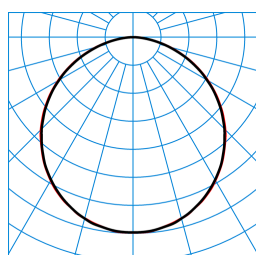
Olisq QWD2 DW 35-830 ET IK + Olisq QWD2 ZDR 1/1 01 TX462188
