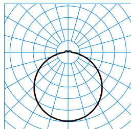
Olisq QWD2 DW 35-830 ET IK + Olisq QWD2 ZDR 1/2 01 TX461741
