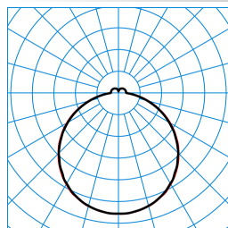
Olisq QWD2 DW 35-830 ET IK TX777164
