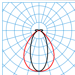
TugraHE+ 12 PN 50-840 ET IP69K 23 TX425171
