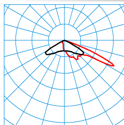
LnPlus 60-AM19L-SLR2/26000-727 24G1 ET (CLO end value) TX390107 DIN 5040: A30 UTE: 1,00 J CEN Flux Code: 28 76 99 100 100 ■ C0 - C180 ■ C90 - C270
