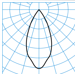
BV G2 3PTD RF-WFL 15-M+F M53 ET 05 TX718728
