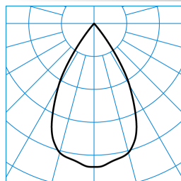
Kalo G2 3P RF-VFL 20-827 M32 ET 01 TX822630
