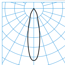
Kalo G2 3P RF-MF-c 30-835 M34 ET 03 TX823005
