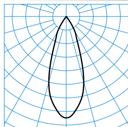
Kalo G2 3P RF-FL-c 30-840 M35 ET 01 TX822767
