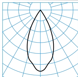
Kalo G2 3P RF-WFL-c 20-EW M48 ET 01 TX821221
