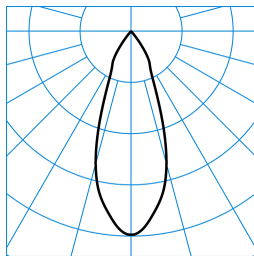
Kalo G2 3P RF-FL 50-840 M35 ETDD 01 TX821352
