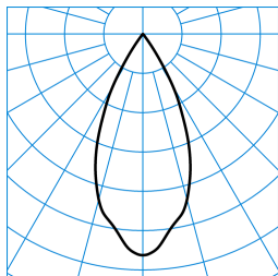
Kalo G2 3P RF-WFL-c 20-M+F M53 ETDD 05 TX824569
