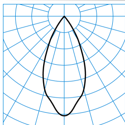
Qui130 G3 RF-WFL 40-827 M32 ET 01 TX828201
