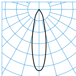
Qui130 G3 RF-MF-c 50-827 M32 ETBLE 05 TX827765
