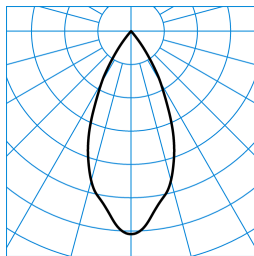
Qui130 G3 RF-WFL 20-835 M34 ET 01 TX827944
