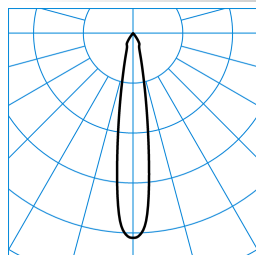
Qui130 G3 RF-SP 30-BF M54 ET 01 TX826389
