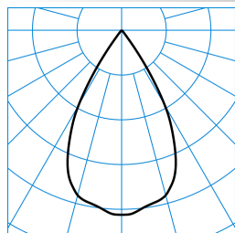
Qui130 G3 RF-VFL-c 30-BF M54 ET 01 TX828345
