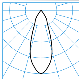
Qui130 G3 RF-FL 15-M+F M53 ET 05 TX826054
