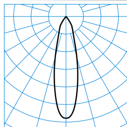
Qui155 G3 RF-MF 40-827 M32 ET 05 TX826595
