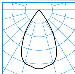
Qui155 G3 RF-VFL 40-830 M33 ET 01 TX828694
