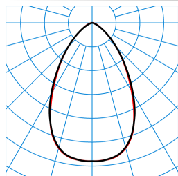
Mirona Fit 2L BS TB 240-840 ETDD TX771132
