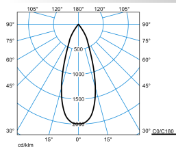
QuiraP G2 RF-FL 50-830 M41 ETDD 01
