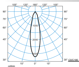
QuiraP G2 RF-MF 70-830 M41 ET 01
