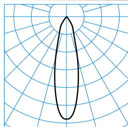
E-Line PRO 78 BV G2 RF-MF 20-830 M33 ET 01 01 TX717141
