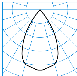
E-Line PRO 78 BV G2 RF-VFL 20-840 M35 ET 01 Blank TX714932
