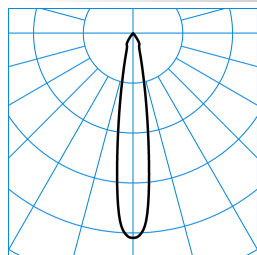
E-Line PRO 78 BV G2 RF-SP 50-840 M35 ET 01 01 TX717255
