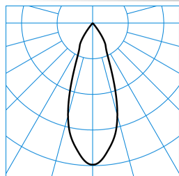
E-Line PRO 78 BV G2 RF-FL 50-840 M35 ET 01 TX714678
