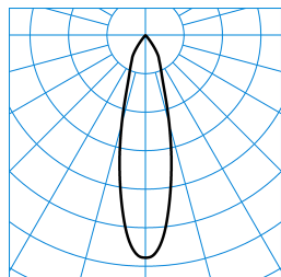
E-Line PRO 78 BV G2 RF-MF 20-EW M48 ET 01 Blank TX717150
