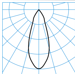
E-Line PRO 78 BV G2 RF-FL 30-827 M32 ET 03 TX716939
