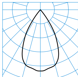
E-Line PRO 78 BV G2 RF-VFL 40-EW M48 ET 03 Blank TX715957
