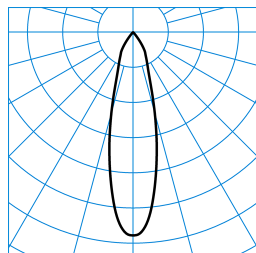
E-Line PRO 78 BV G2 RF-MF 30-827 M32 ET 05 Blank TX716278
