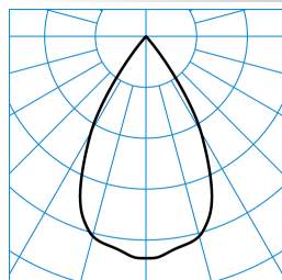
E-Line PRO 78 BV G2 RF-VFL 50-835 M34 ET 05 TX716507
