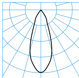
E-Line PRO 78 BV G2 RF-FL 40-840 M35 ET 05 Blank TX716206
