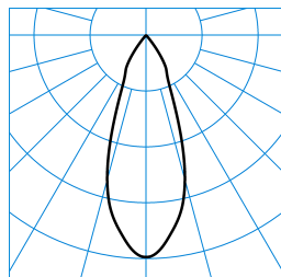
E-Line PRO 78 BV G2 RF-FL 30-BF M54 ET 05 Blank TX716175
