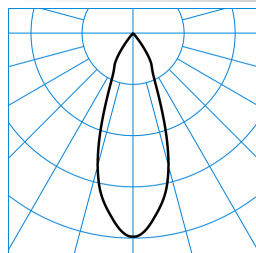
E-Line PRO 78 BV G2 RF-FL 30-BF M54 ET 05 TX716173
