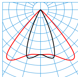
E-Line PRO 78 Grado WRS-DF84 40-830 M41 ET 01 Blank TX717368
