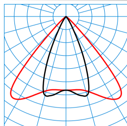
E-Line PRO 78 Grado WRS-DF84 40-830 M41 ET 01 01 TX715003
