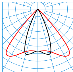
E-Line PRO 78 Grado WRS-DF84 40-830 M41 ET 03 Blank TX715675
