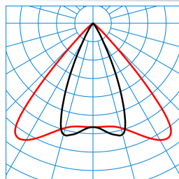
E-Line PRO 78 Grado WRS-DF84 40-840 M43 ET 05 TX716641
