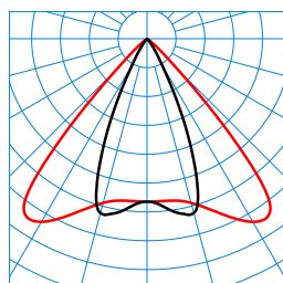
E-Line PRO 78 Grado WRS-DF84 50-840 M43 ETDD 05 Blank TX716673
