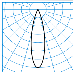
E-Line PRO 78 Lentyp L-MF 20-830 M33 ET 01 TX717434
