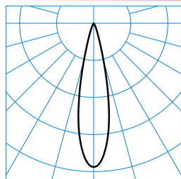
E-Line PRO 78 Lentyp L-SP 20-EC M39 ET 01 TX717490
