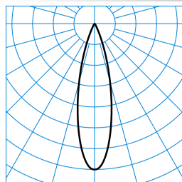
E-Line PRO 78 Lentyp L-MF 40-827 M32 ET 03 TX715767
