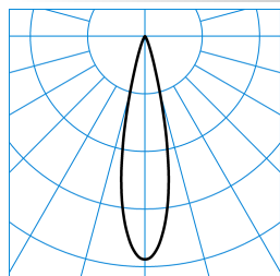
E-Line PRO 78 Lentyp L-SP 20-840 M35 ET 03 TX715786
