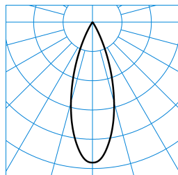
E-Line PRO 78 Lentyp L-FL 20-827 M32 ET 05 Blank TX716686
