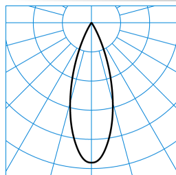
E-Line PRO 78 Lentyp L-FL 20-835 M34 ET 05 TX716688
