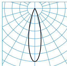
E-Line PRO 78 Lentyp L-MF 30-835 M34 ET 05 Blank TX716780
