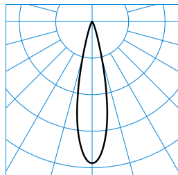
E-Line PRO 78 Lentyp L-SP 40-835 M34 ET 05 TX716876
