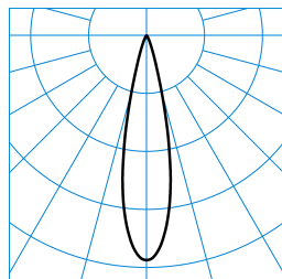
E-Line PRO 78 Lentyp L-SP 20-EW M48 ET 05 Blank TX715057
