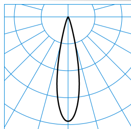
E-Line PRO 78 Lentyp L-SP 20-EW M48 ET 05 TX716841
