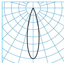
E-Line PRO 78 Lentyp L-MF 40-EW M48 ET 05 Blank TX716823
