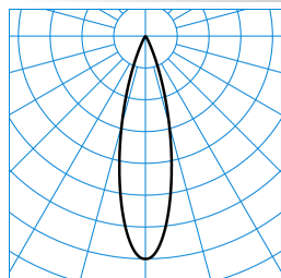
E-Line PRO 78 Lentyp L-MF 40-EW M48 ET 05 TX716822
