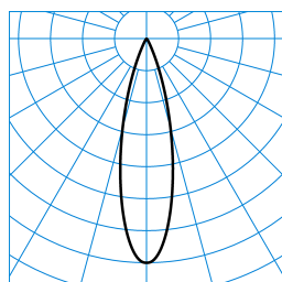
E-Line PRO 78 Lentyp L-MF 40-840 M35 ETDD 03 Blank TX716073
